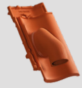
Ceramiczna dachówka przelotowa do systemu baterii solarnych
